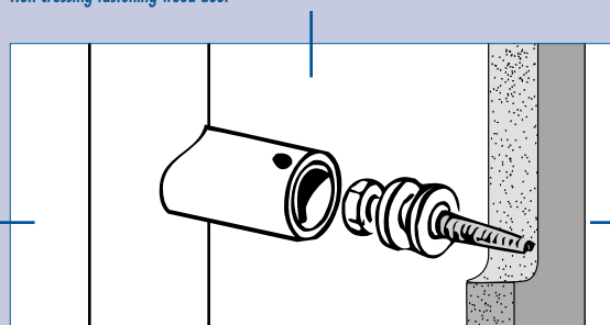
Fixation non traversante sur porte bois Non-crossing fastening wood door
