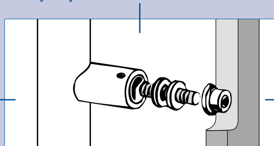
Fixation non traversante sur porte alu avec insert Non-crossing fastening on aluminium with insert
