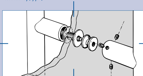
Montage double (par paire) Double assembly (by pair)
